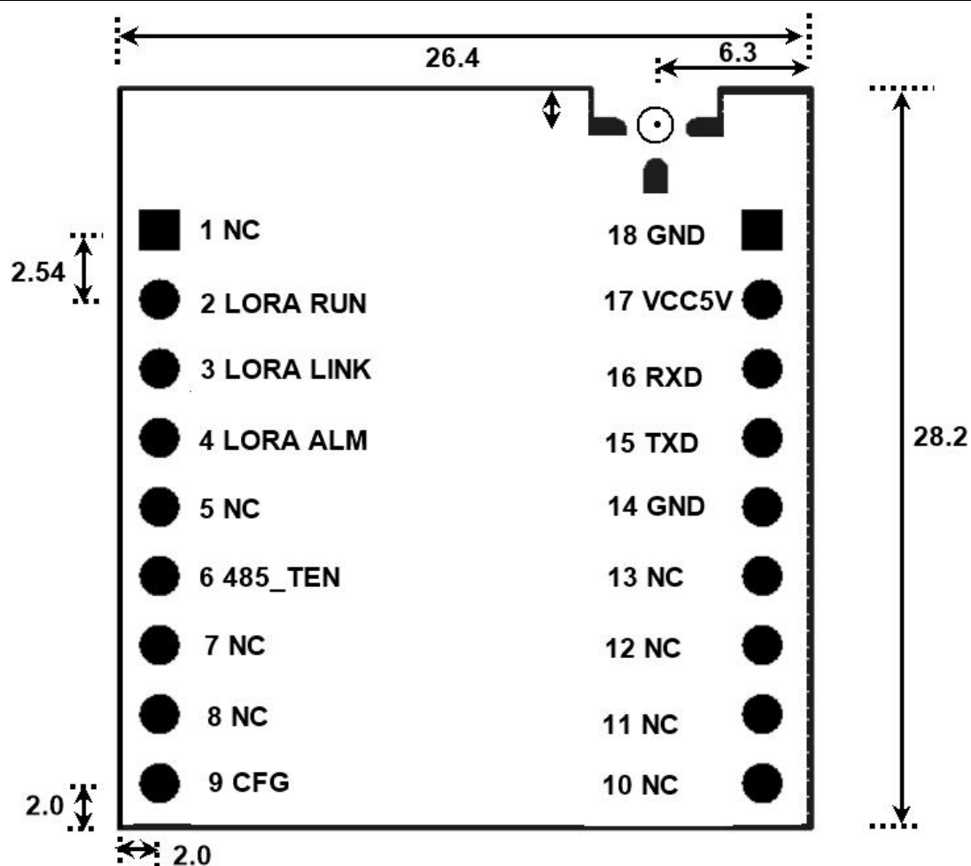
图 4 ZLSN9700C 正面引脚图
